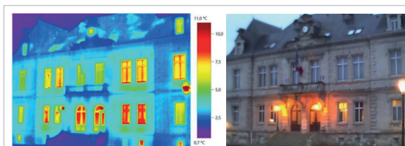
Thermographie de la Mairie de Creil
